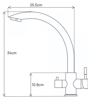
WDF-LT1803-SS
